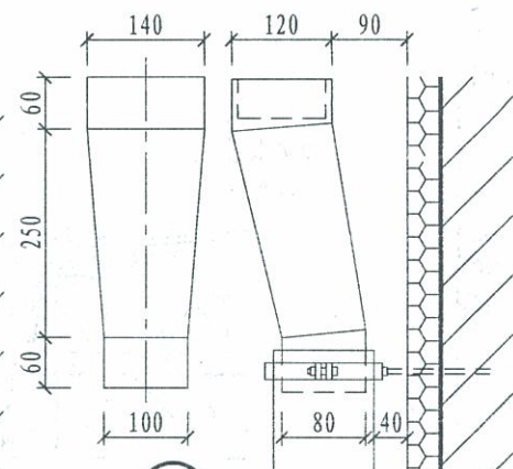
④ 方雨水接口
