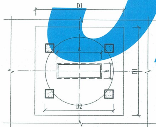
B-B自力式风帽平面图
