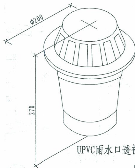
⑦ UPVC雨水口
