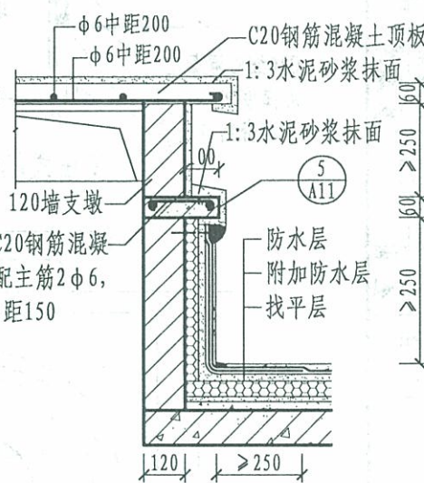
① 烟囱、通风道出屋面节点
