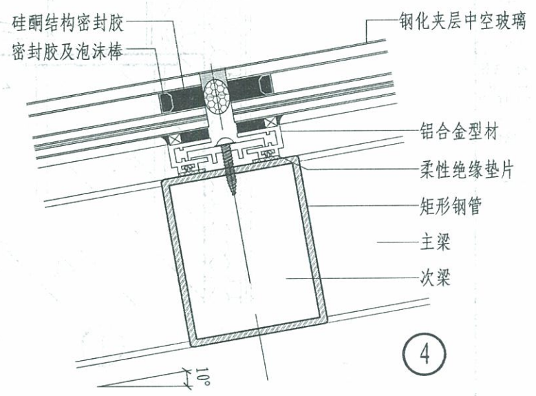
半隐框玻璃采光顶节点 (一)
