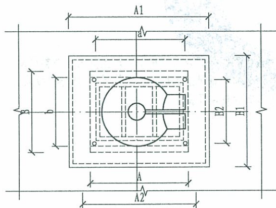
C-C止回式风帽平面图
