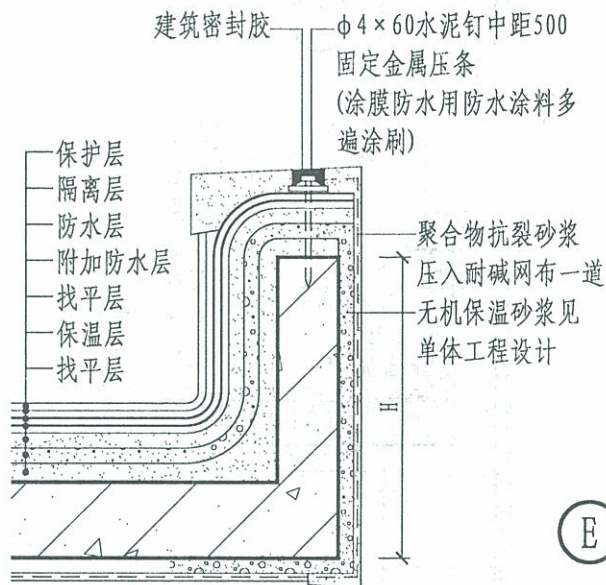
卷材、涂膜防水屋面 节点详图 (一)
