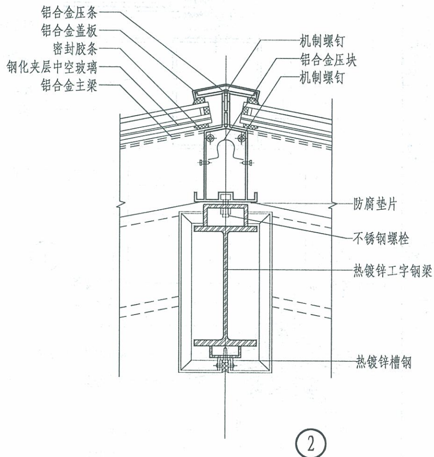
半隐框玻璃采光顶节点（二）
