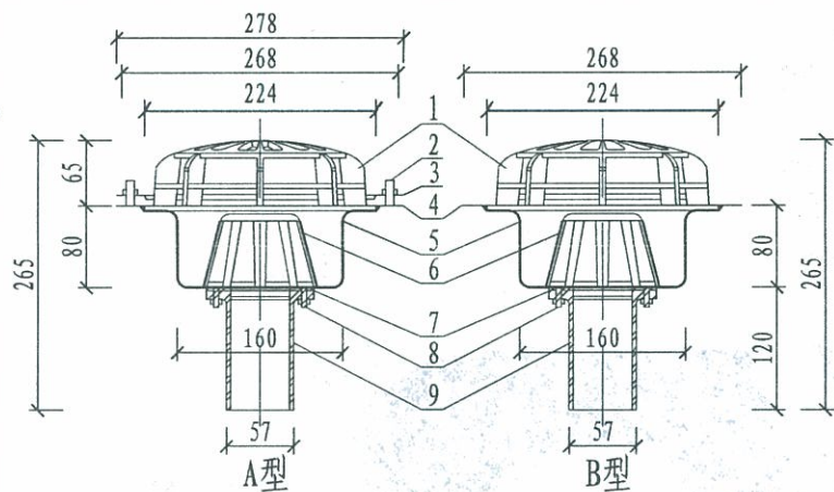
① YG50型虹吸式雨水斗
