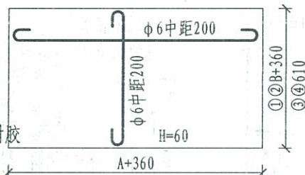
顶板配筋
