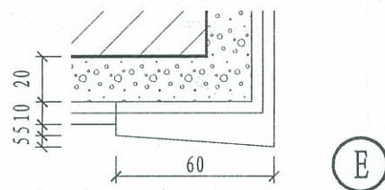
卷材、涂膜防水屋面 檐口详图
