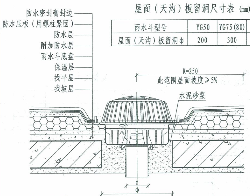
1 虹吸式雨水斗在屋面 (天沟) 板上安装 (YG50、75、80、100A型)
