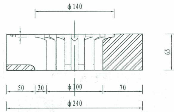
2-2剖面图
