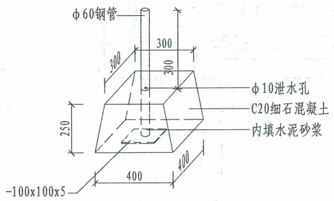
屋面旗杆座透视图
