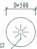
雨水口附加防水层叉面裁剪图
