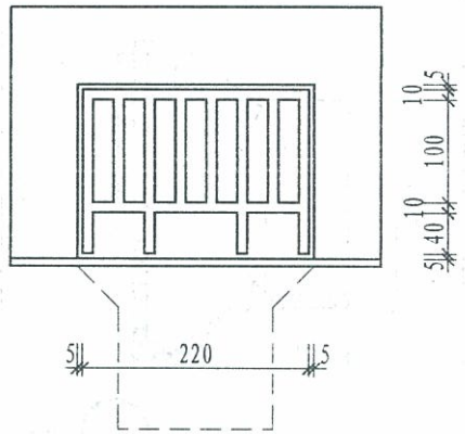
立面
