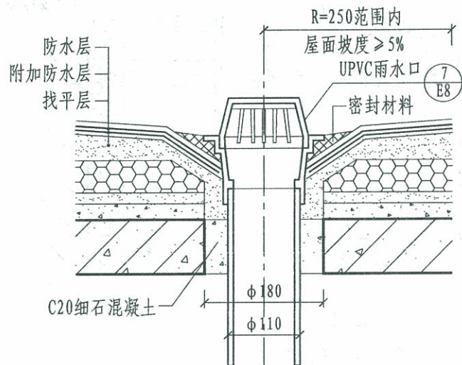
⑥ 内排水UPVC雨水口
