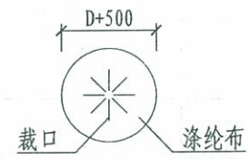
2 附加防水层叉面裁剪图
