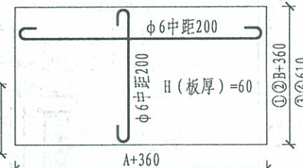
顶板构造
