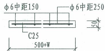
GB-1配筋图
