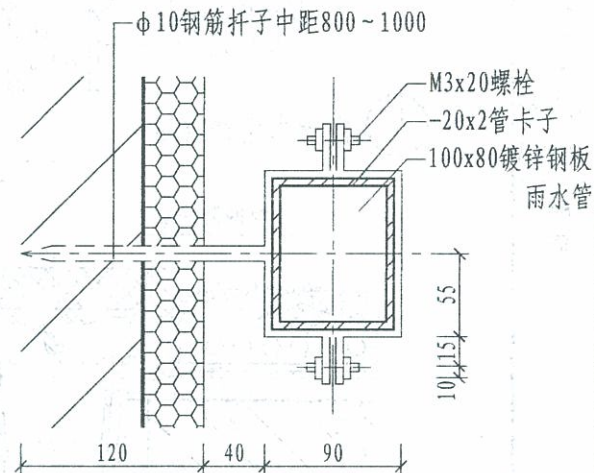
⑤ 方雨水管及卡子
