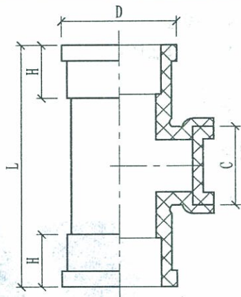
② UPVC检查口
