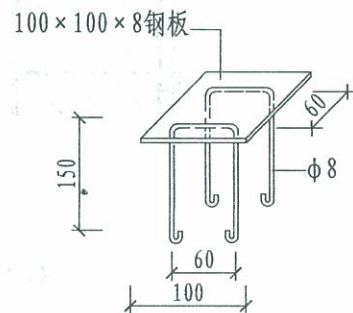
④ 预埋铁件
