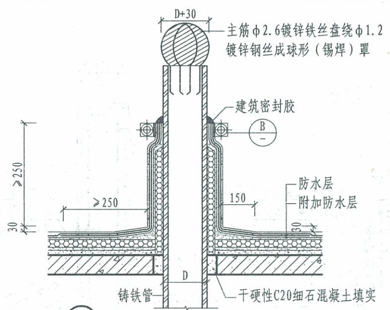
① 铸铁管出屋面
