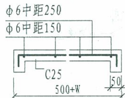
GB-1配筋图 (板长1000)
