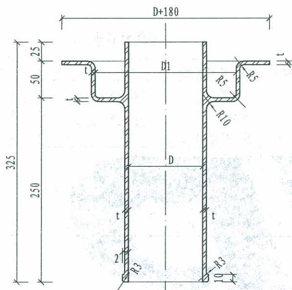
1-1剖面图
