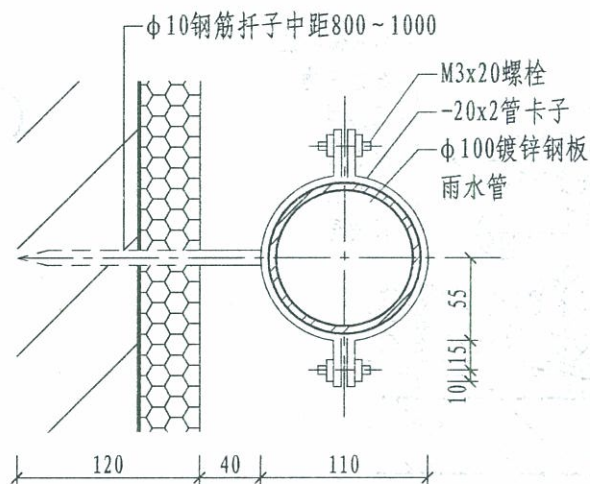
④ 圆雨水管及卡子
