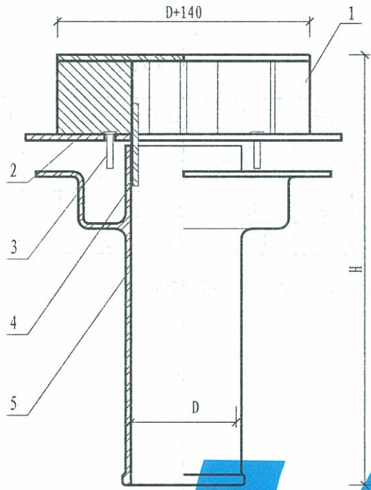
① 铸铁短管雨水斗总装配图
