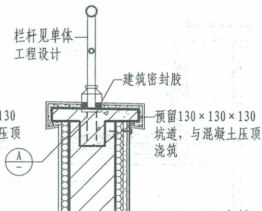
③ 栏杆
