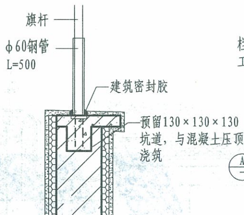
② 旗杆
