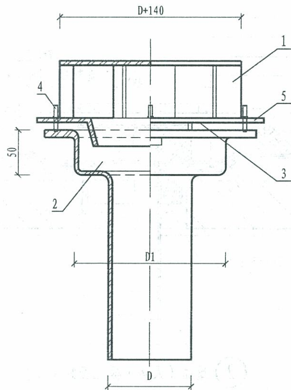
① 87改进型雨水斗装配图
