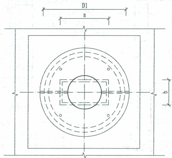
A-A变压式风帽平面图
