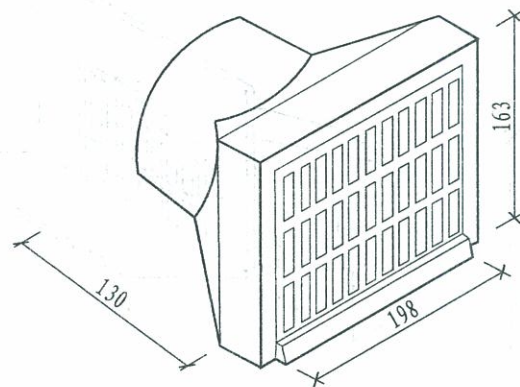
UPVC外雨水口透视
