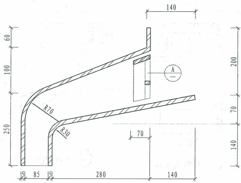
1-1剖面
