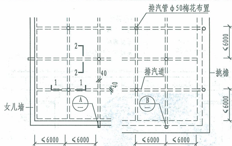
排汽道、排汽管平面布置图
