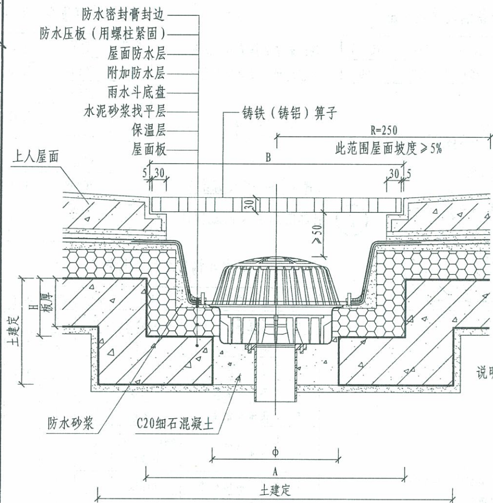
① 上人屋面YG(A型)虹吸式雨水斗安装 (屋面板局部下凹)
