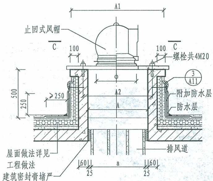
止回式风帽出屋面做法
