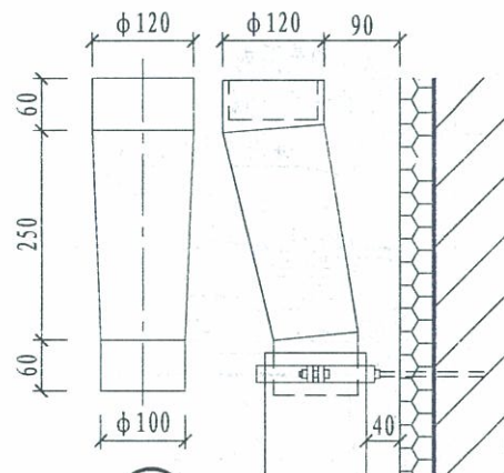
③ 圆雨水接口
