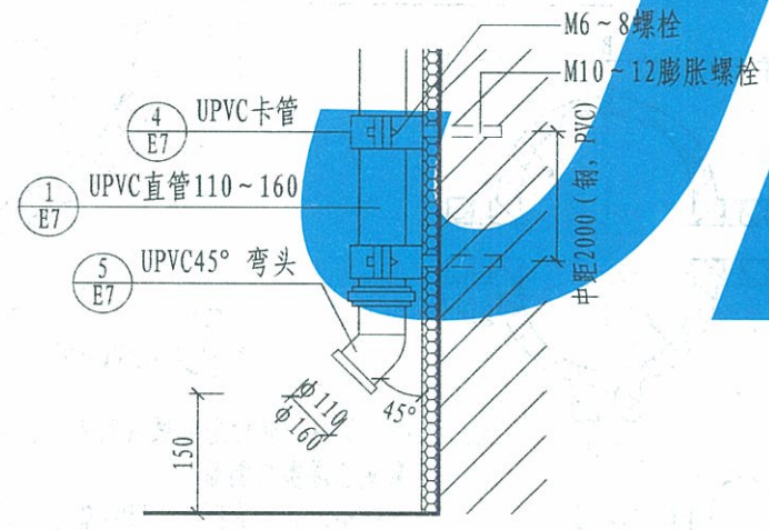
② 外排UPVC管底出水口
