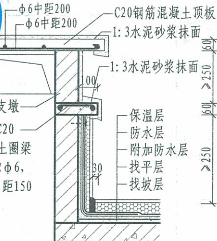
顶板配筋
