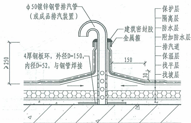
1-1
