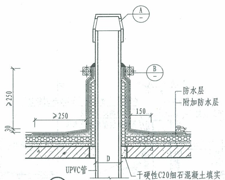
② UPVC管出屋面
