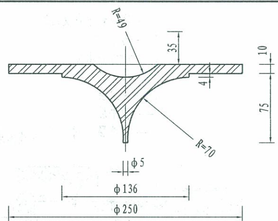
1-1剖面图
