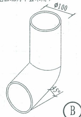
外排镀锌钢板管底方(圆)出水口 注: 镀锌钢板0.6厚。
