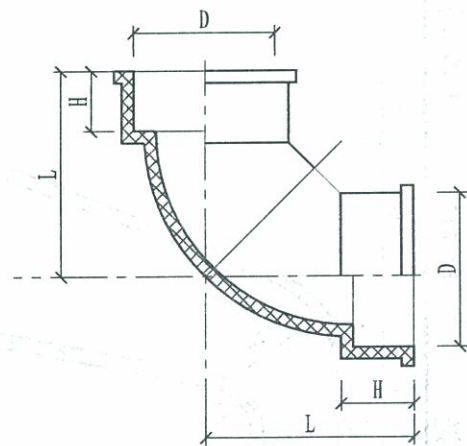
⑧ UPVC90° 弯头
