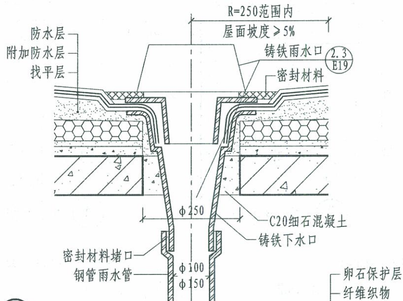
⑤ 内排水铸铁雨水口
