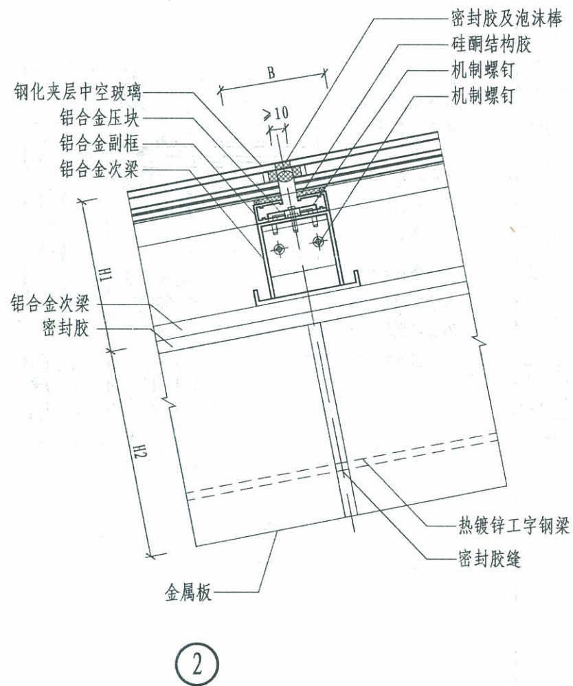
隐框双坡采光顶节点（三）
