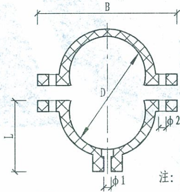
④ UPVC卡管
