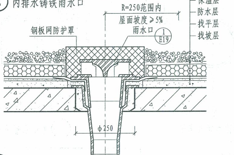
⑦ 倒置式屋面内排水雨水口
