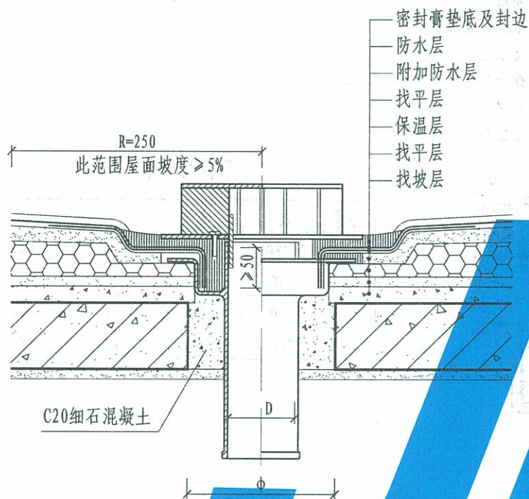
① 屋面(天沟)板上安装图
