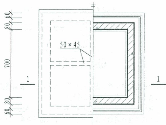
① 屋面检修孔平面
