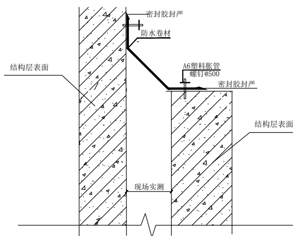
外墙变形缝做法 (错台)
