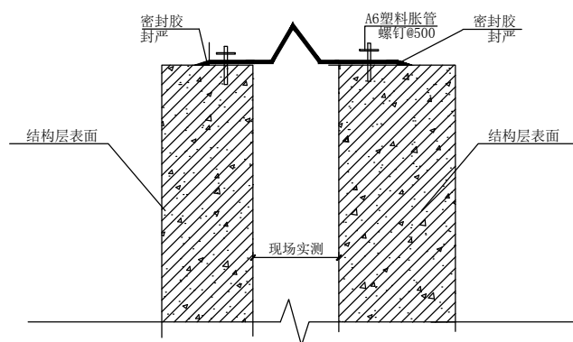
外墙变形缝做法 (平)
